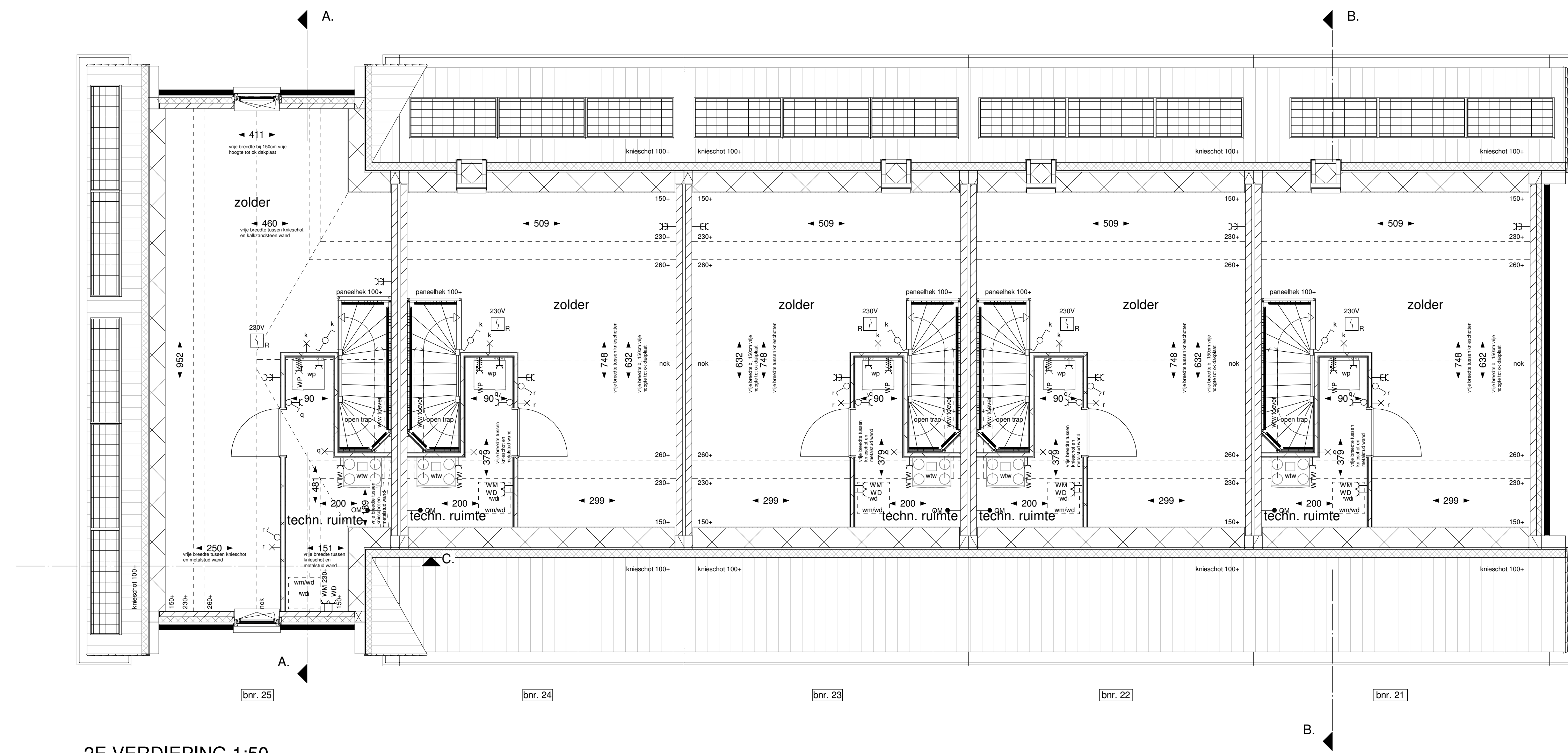
2E VERDIEPING 1:50
