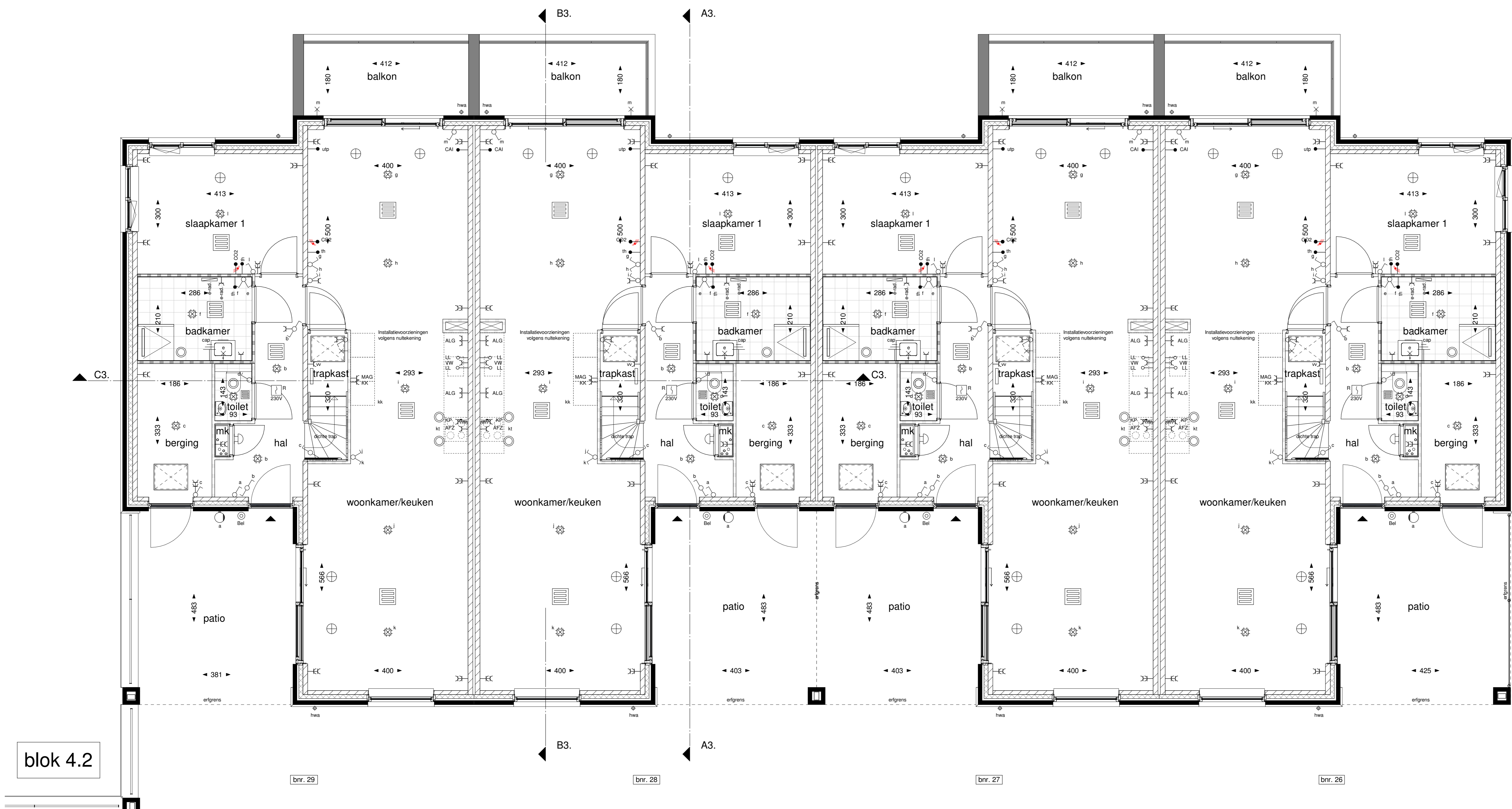
BEGANE GROND 1:50
